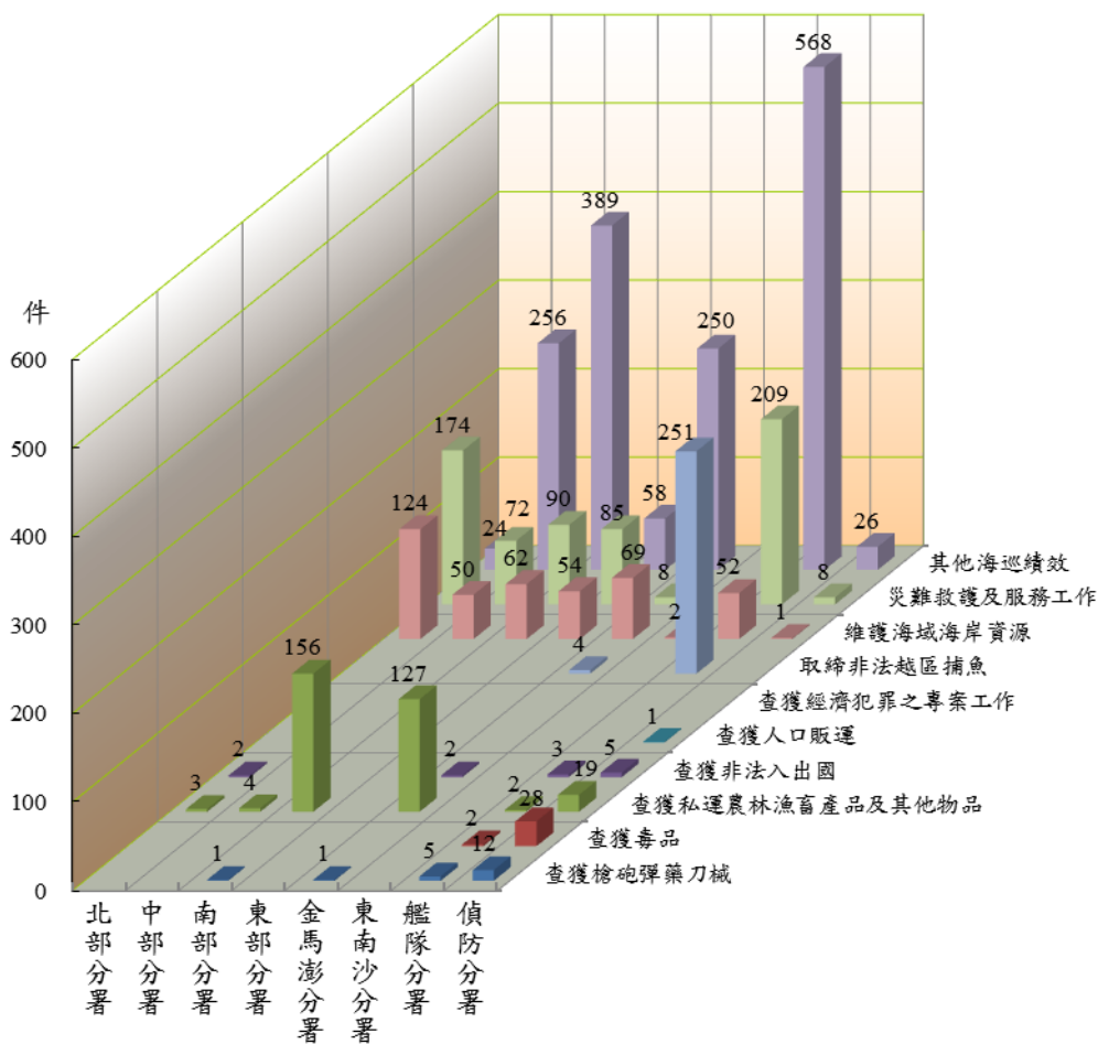
圖11 113年1-6月各分署海巡績效案件數統計
